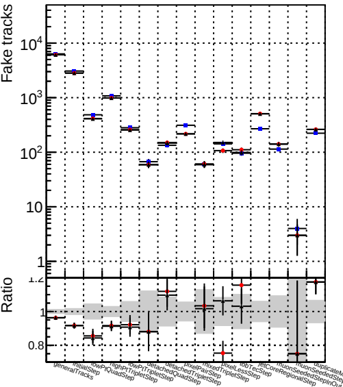
Number —■— DQMstep3_SMS_CKF —●— DQMstep3_SMS_default —★— DQMstep3_SMS_ckfPixelLess
