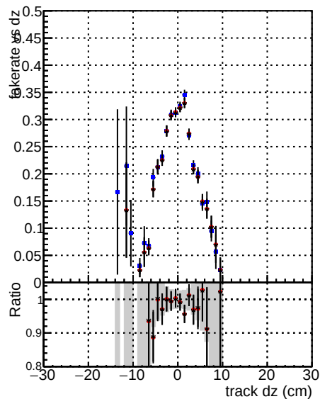
Fake rate vs dz — DOMstep3 SMS CKF — default — DOMstep3 SMS CKFPixelLess
