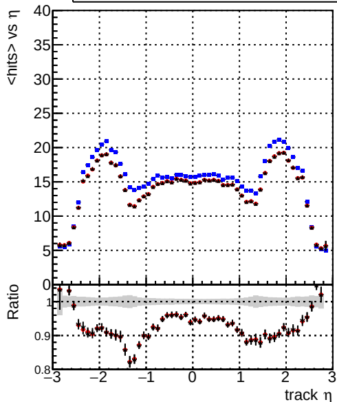
mean hit — DQMstep3_SMS_CKF — DQMstep3_SMS_default — DQMstep3_SMS_ckptPixelLess
