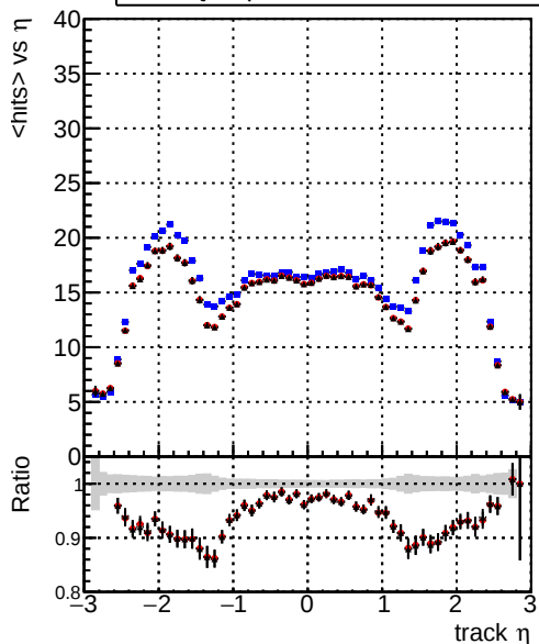
mean hit — DQMstep3_SMS_CKF — DQMstep3_SMS_default — DQMstep3_SMS_ckfPixelLess
