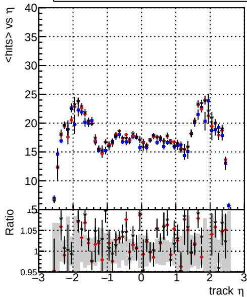
mean hit — DQMstep3_SMS_CKF — DQMstep3_SMS_default — DQMstep3_SMS_ckptPixelLess
