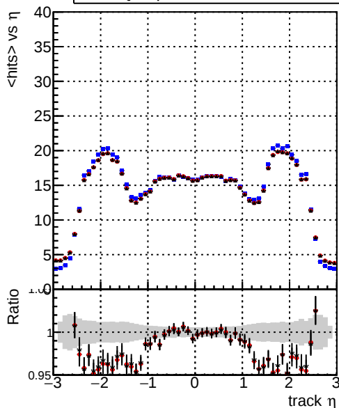
mean hit — DQMstep3_SMS_CKF — DQMstep3_SMS_default — DQMstep3_SMS_ckfPixelLess
