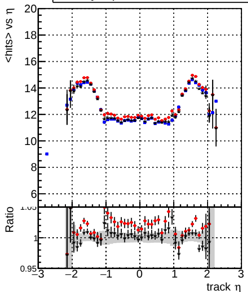
mean hits vs \eta — DQMstep3_SMS_CKF — DQMstep3_SMS_default — DQMstep3_SMS_ckfPixelLess
