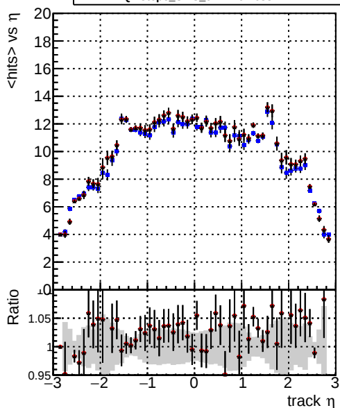
mean hits vs \eta — DQMstep3_SMS_CKF — DQMstep3_SMS_default — DQMstep3_SMS_ckfPixelLess
