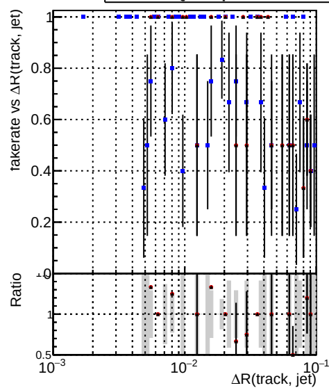
—●— DQMstep3 SMS CKF —●— DQMstep3 SMS default —●— DQMstep3 SMS_ckfPixelLess
