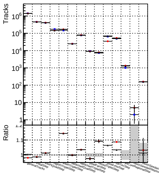
Number of tracks vs collection DQMstep3_SMS_CKF DQMstep3_SMS_default DQMstep3_SMS_ckfPixelLess
