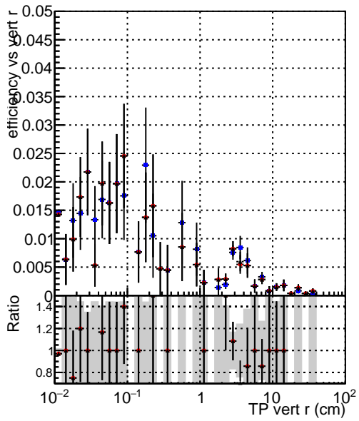
—●— DQMstep3_SMS_CKF —●— DQMstep3_SMS_default —●— DQMstep3_SMS_ckfPixelLess
