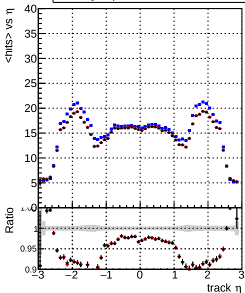
mean hits — DQMstep3_SMS_CKF — DQMstep3_SMS_default — DQMstep3_SMS_ckptPixelLess
