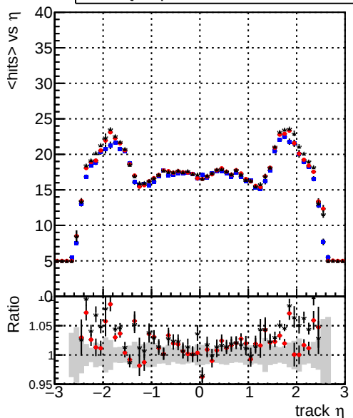
mean hit — DQMstep3_SMS_CKF — DQMstep3_SMS_default — DQMstep3_SMS_ckptPixelLess
