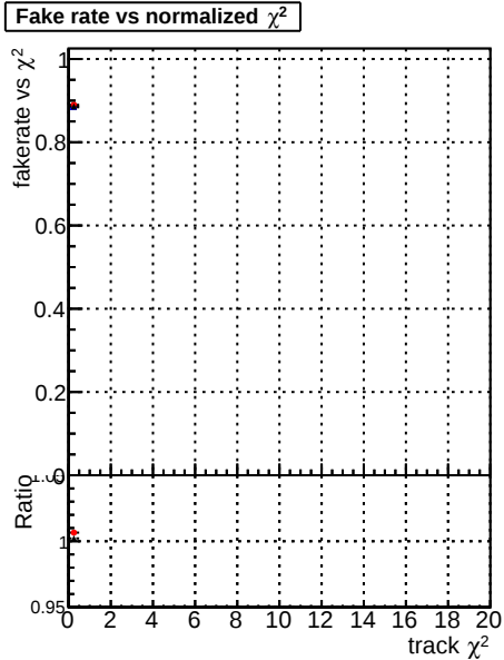
Fake rate vs. \chi^2 DOMstep3 SMS CKF DOMstep3 SMS default DOMstep3 SMS defaultNEWT
