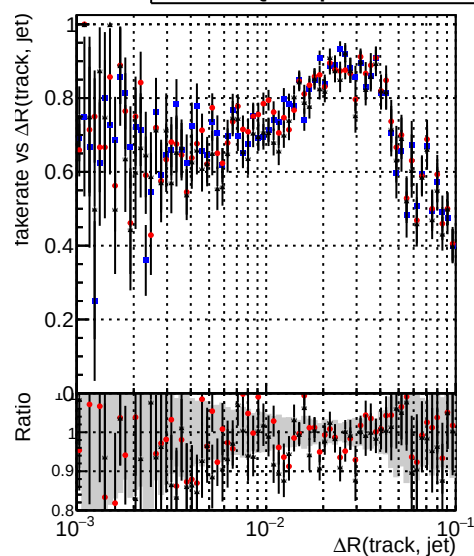
—●— DQMstep3 SMS CKF —●— DQMstep3 SMS default —●— DQMstep3 SMS defaultNEWT
