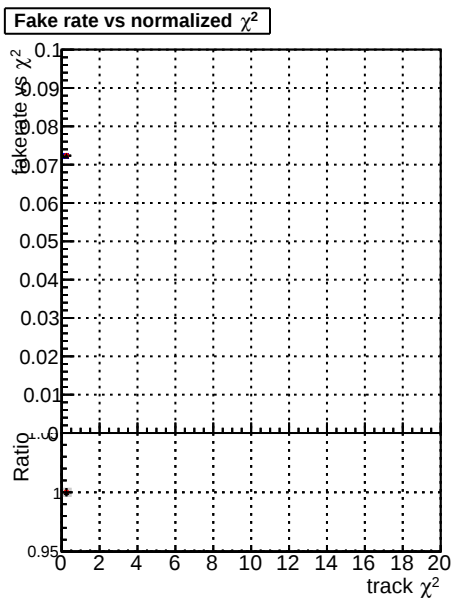
Fake rate vs. DOMstep3 SMS CKF DOMstep3 SMS default DOMstep3 SMS defaultNEWT
