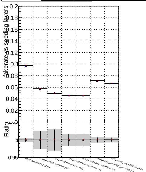
Fake rate vs. DOMstep3 SMS CKF DOMstep3 SMS default DOMstep3 SMS defaultNEWT
