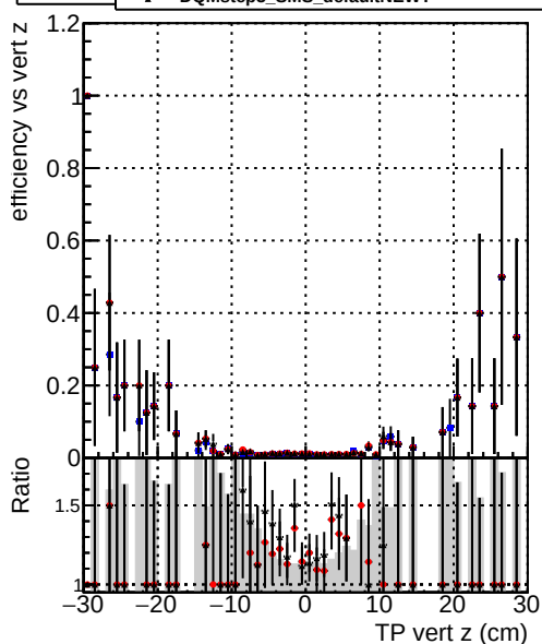
Efficiency —●— DQMstep3_SMS_default —★— DQMstep3_SMS_defaultNEWT
