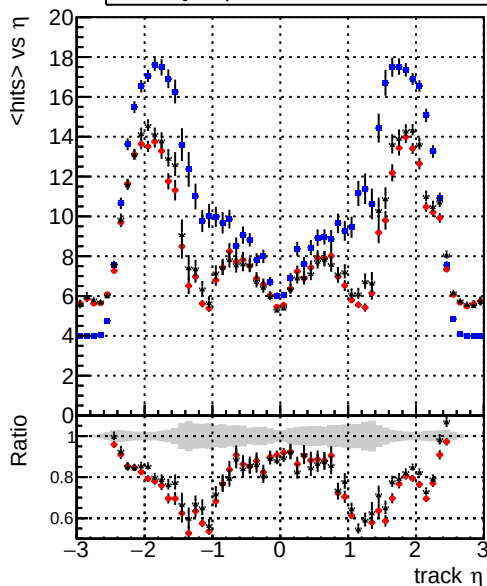
mean hit — DQMstep3_SMS_CKF — DQMstep3_SMS_default — DQMstep3_SMS_defaultNEWT
