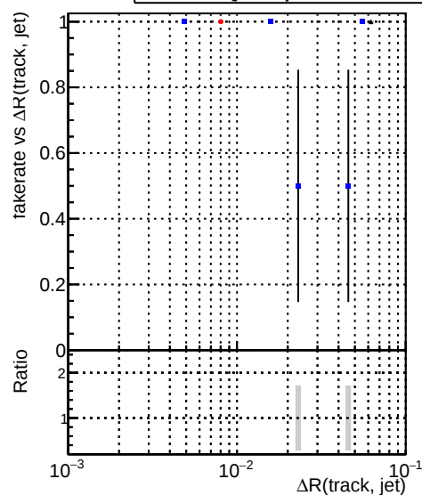
—●— DQMstep3_SMS_CKF —●— DQMstep3_SMS_default —●— DQMstep3_SMS_defaultNEWT
