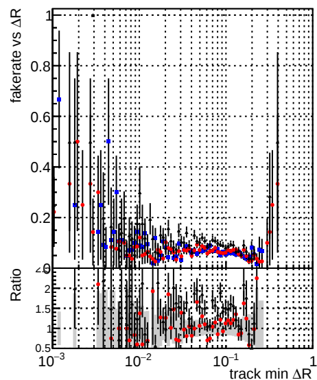
—●— DQMstep3_SMS_CKF —●— DQMstep3_SMS_default —●— DQMstep3_SMS_defaultNEWT
