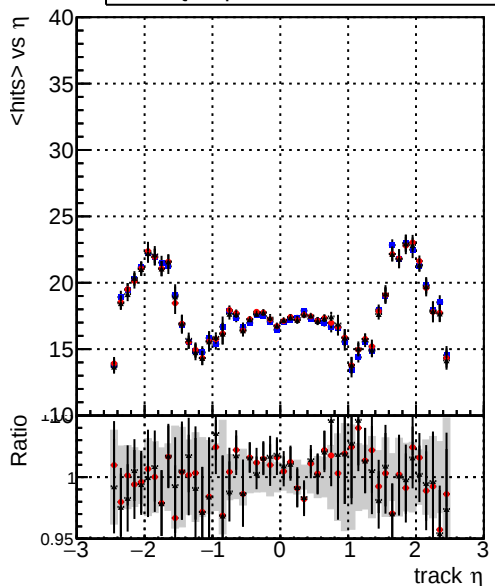
DQMstep3_SMS_CKF DQMstep3_SMS_default DQMstep3_SMS_defaultNEWT mean hits
