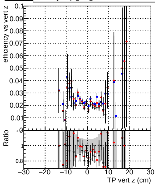
Efficiency vs vert z —•— DQMstep3_SMS_CKF —•— DQMstep3_SMS_default —•— DQMstep3_SMS_defaultNEWT
