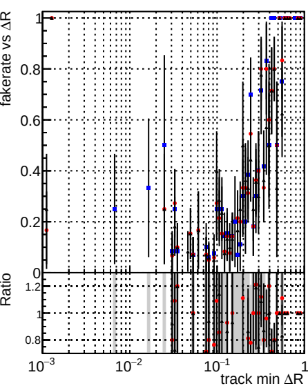
Fake rate vs \Delta R(\text{track, jet}) DQMstep3 SMS CKF DQMstep3 SMS default DQMstep3 SMS defaultNEWT
