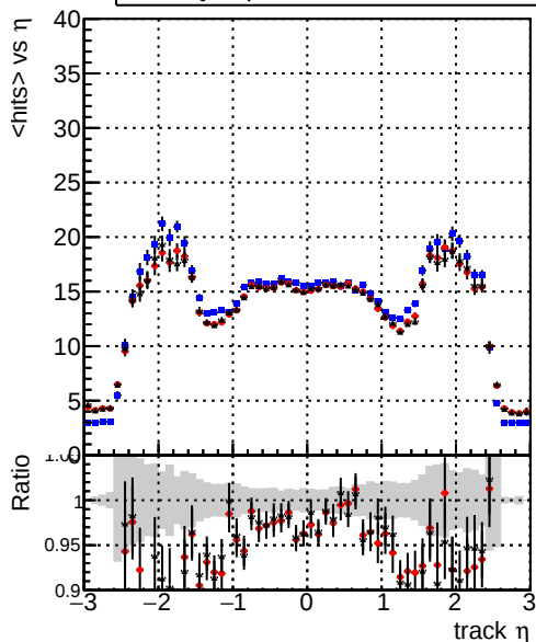
mean hits — DQMstep3_SMS_CKF — DQMstep3_SMS_default — DQMstep3_SMS_defaultNEWT
