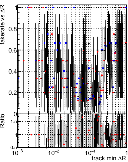
Fake rate vs —●— DQMstep3_SMS_CKF —●— DQMstep3_SMS_default —●— DQMstep3_SMS_defaultNEWT
