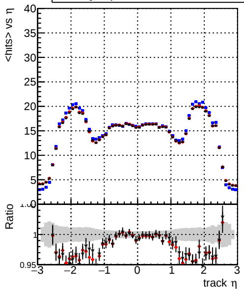
mean hit — DQMstep3_SMS_CKF — DQMstep3_SMS_default — DQMstep3_SMS_defaultNEWT
