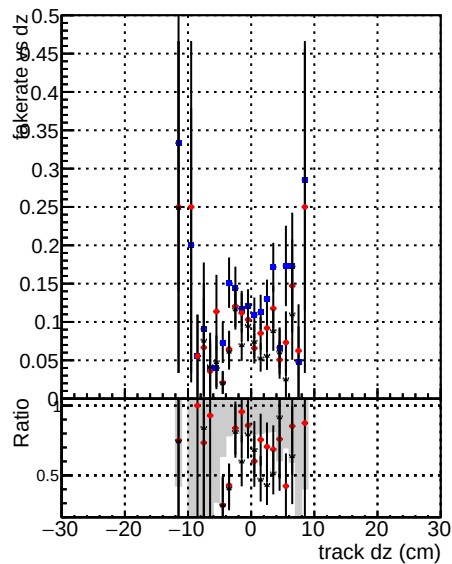
Fake rate vs dz DOMstep3 SMS CKF DOMstep3 SMS default DOMstep3 SMS default NEWT
