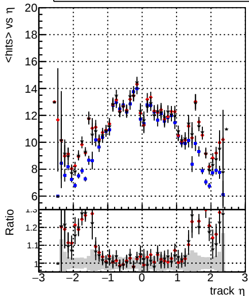
DQMstep3_SMS_CKF DQMstep3_SMS_default DQMstep3_SMS_defaultNEWT mean hits
