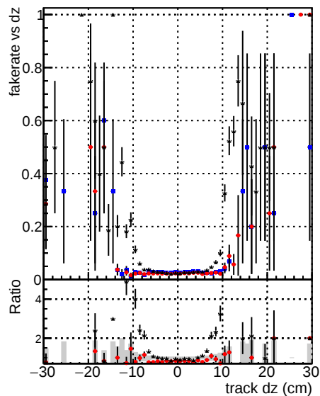
—•— DOMstep3 SMS CKF —•— DOMstep3 SMS default —•— DOMstep3 SMS defaultNEWT
