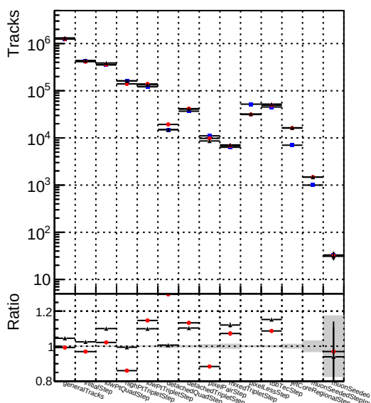
Number —■— DQMstep3_SMS_CKF —●— DQMstep3_SMS_default —▲— DQMstep3_SMS_defaultNEWT
