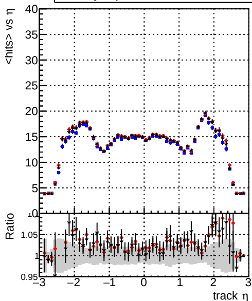
mean hits vs \eta — DQMstep3_SMS_CKF — DQMstep3_SMS_default — DQMstep3_SMS_defaultNEWT
