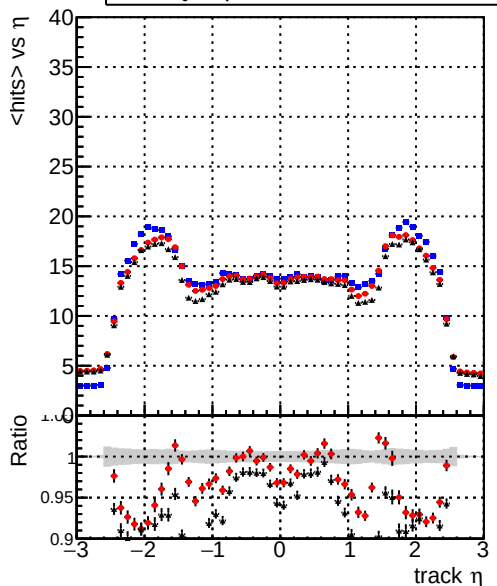
mean hits — DQMstep3_SMS_CKF — DQMstep3_SMS_default — DQMstep3_SMS_defaultNEWT
