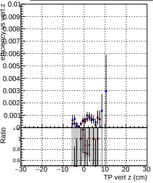
Efficiency vs TP vert z (cm) Legend: DQMstep3_QCD_CKF (blue stars) DQMstep3_QCD_default (red dots) DQMstep3_QCD_ckfPixelLess (black crosses)
