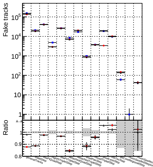
Number Legend 1 DQMstep3_QCD_default 2 DQMstep3_QCD_ckfPixelLess
