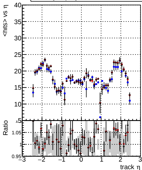
— DQMstep3_QCD_CKF — DQMstep3_QCD_default — DQMstep3_QCD_ckfPixelLess mean hits
