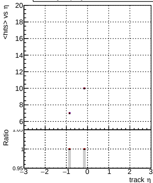
mean hit — DQMstep3_QCD_CKF — DQMstep3_QCD_default — DQMstep3_QCD_ckfPixelLess
