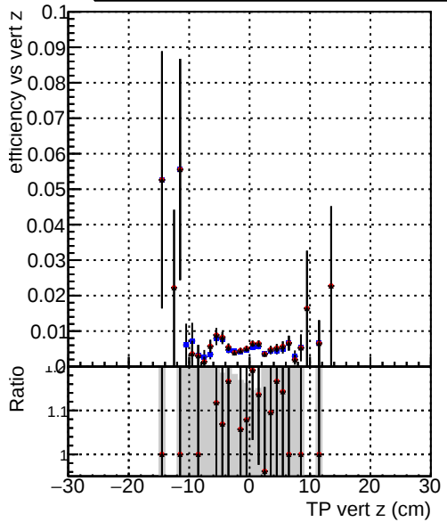
Efficiency vs. TP vert z (cm) —●— DQMstep3_QCD_CKF —●— DQMstep3_QCD_default —●— DQMstep3_QCD_ckfPixelLess
