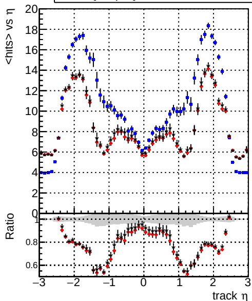
mean hits vs \eta — DQMstep3_QCD_CKF — DQMstep3_QCD_default — DQMstep3_QCD_ckfPixelLess
