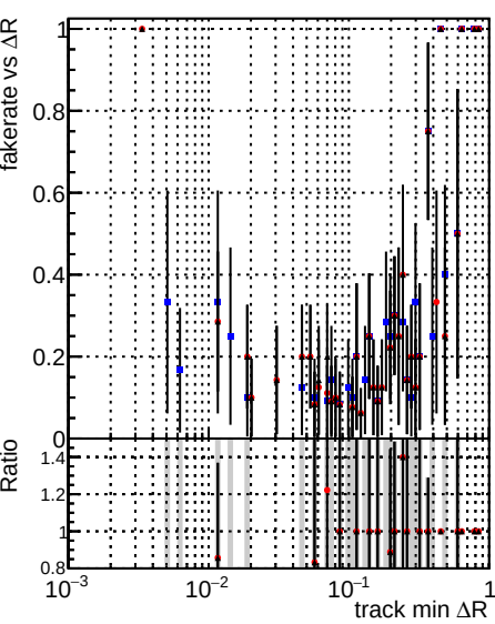
Legend: DQMstep3_QCD_CKF (blue dots), DQMstep3_QCD_default (red dots), DQMstep3_QCD_ckfPixelLess (black dots)
