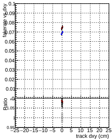
— DOMstep3 OCB GKF — DOMstep3 OCB default — DOMstep3 OCB CRPixelLess
