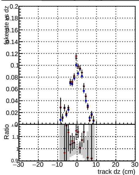
— DOMstep3 OCB GKF — DOMstep3 OCB default — DOMstep3 OCB CRPixelLess
