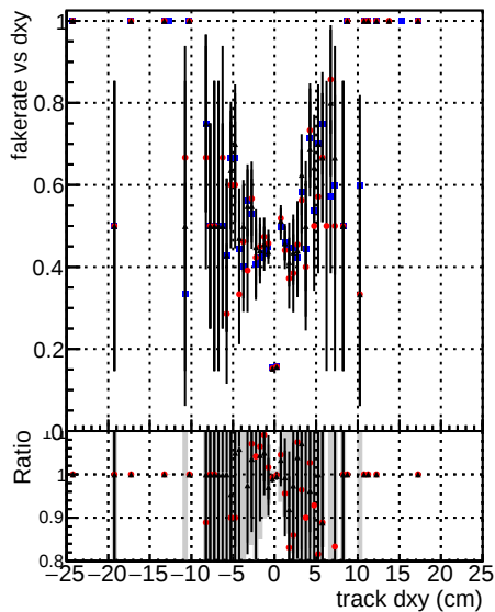
— DOMstep3 OCB CKF — DOMstep3 OCB default — DOMstep3 OCB CKPixelLess
