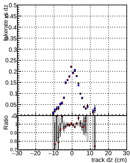
— DOMstep3 OCB CKF — DOMstep3 OCB default — DOMstep3 OCB CKPixelLess
