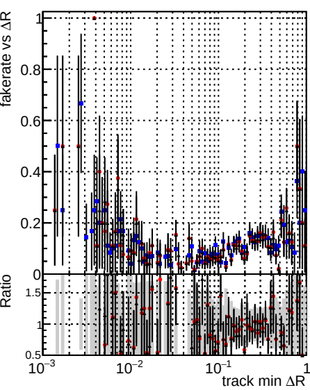
Fake rate vs \Delta R(\text{track, jet}) DQMstep3_QCD_CKF DQMstep3_QCD_default DQMstep3_QCD_ckfPixelLess
