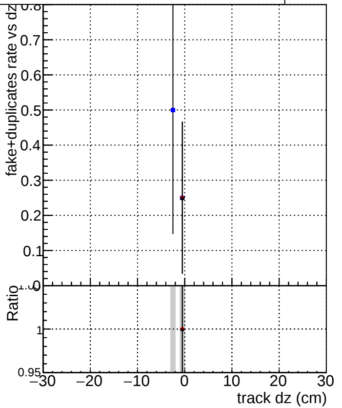
DQMstep3_QCD_CKF DQMstep3_QCD_default DQMstep3_QCD_ckfPixelLess
