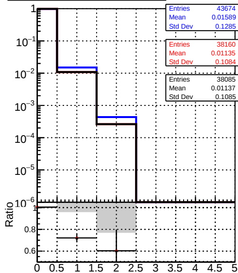
mean hits — DQMstep3_QCD_CKF — DQMstep3_QCD_default — DQMstep3_QCD_ckfPixelLess
