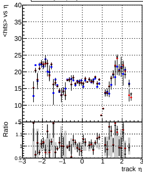
mean hit — DQMstep3_QCD_CKF — DQMstep3_QCD_default — DQMstep3_QCD_ckfPixelLess
