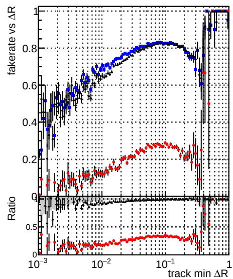
—●— DQMstep3_QCD_CKF —●— DQMstep3_QCD_default —●— DQMstep3_QCD_ckfPixelLess
