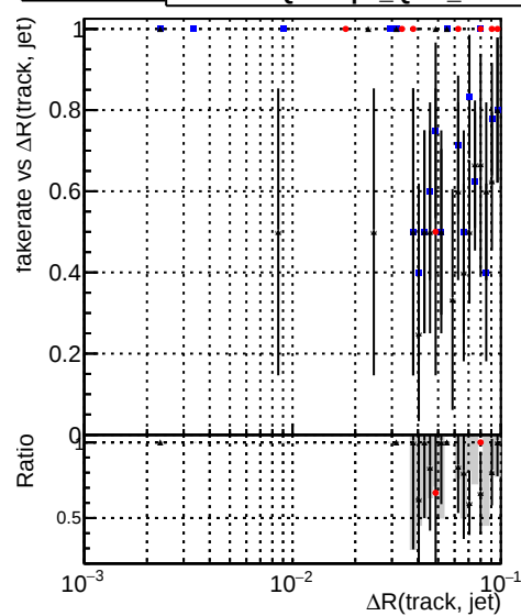
—●— DQMstep3_QCD_CKF —●— DQMstep3_QCD_default —●— DQMstep3_QCD_ckfPixelLess
