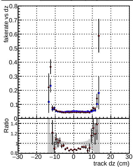
DOMstep3 OCB CKF DOMstep3 OCB default DOMstep3 OCB CRPixelLess
