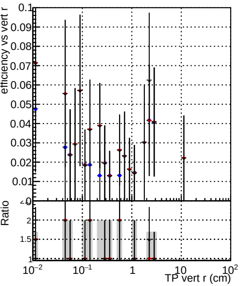
Efficiency vs TP vert r (cm) Legend: DQMstep3_QCD_CKF (blue dots) DQMstep3_QCD_default (red dots) DQMstep3_QCD_ckfPixelLess (black dots)
