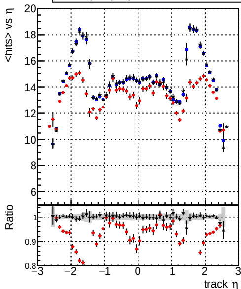
mean hits — DQMstep3_QCD_CKF — DQMstep3_QCD_default — DQMstep3_QCD_ckfPixelLess
