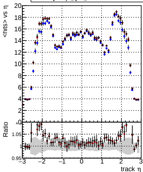
mean hits vs \eta DQMstep3_QCD_CKF DQMstep3_QCD_default DQMstep3_QCD_ckfPixelLess
