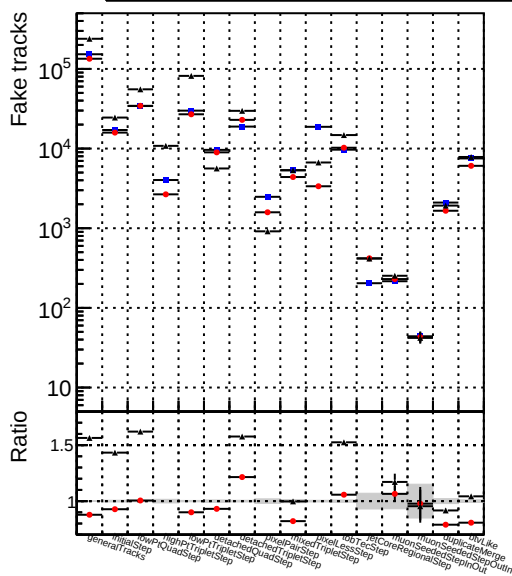
Number Legend 1 DQMstep3_QCD_default 2 DOMstep3_QCD_defaultNEW
